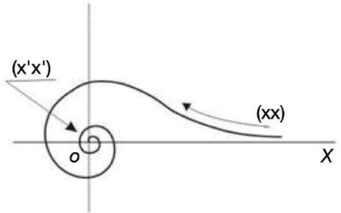
Lituus \rho^2 \theta = a^2
